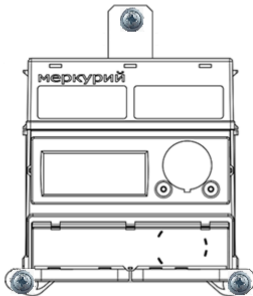
Рисунок 6.2 – Крепеж счетчика на плоскую поверхность
