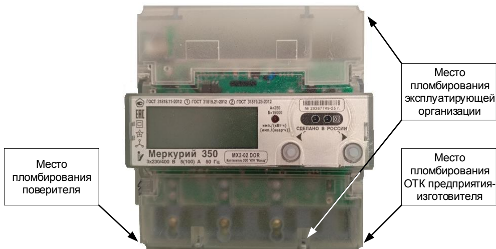
Рисунок 4.3 – Вид счетчика Меркурий 350MX с указанием мест пломбирования и нанесения знака поверки
