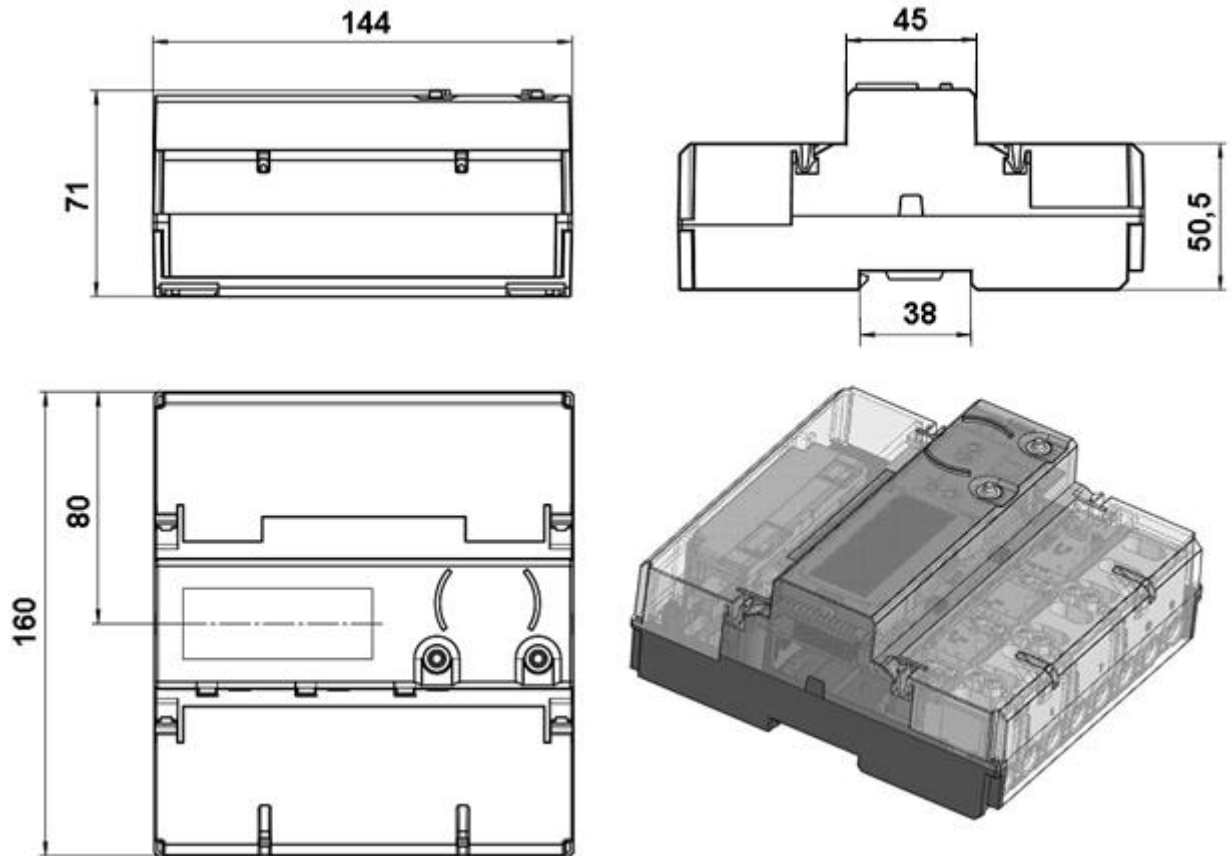
Рисунок А.2 – Габаритный чертеж счетчика Меркурий 350Х
