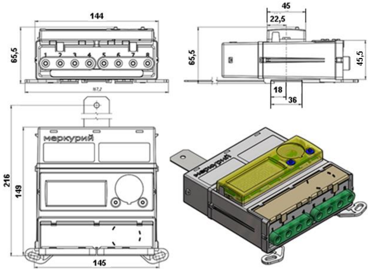
Рисунок А.1 – Габаритный чертеж счетчиков Меркурий 350М, Меркурий 350
