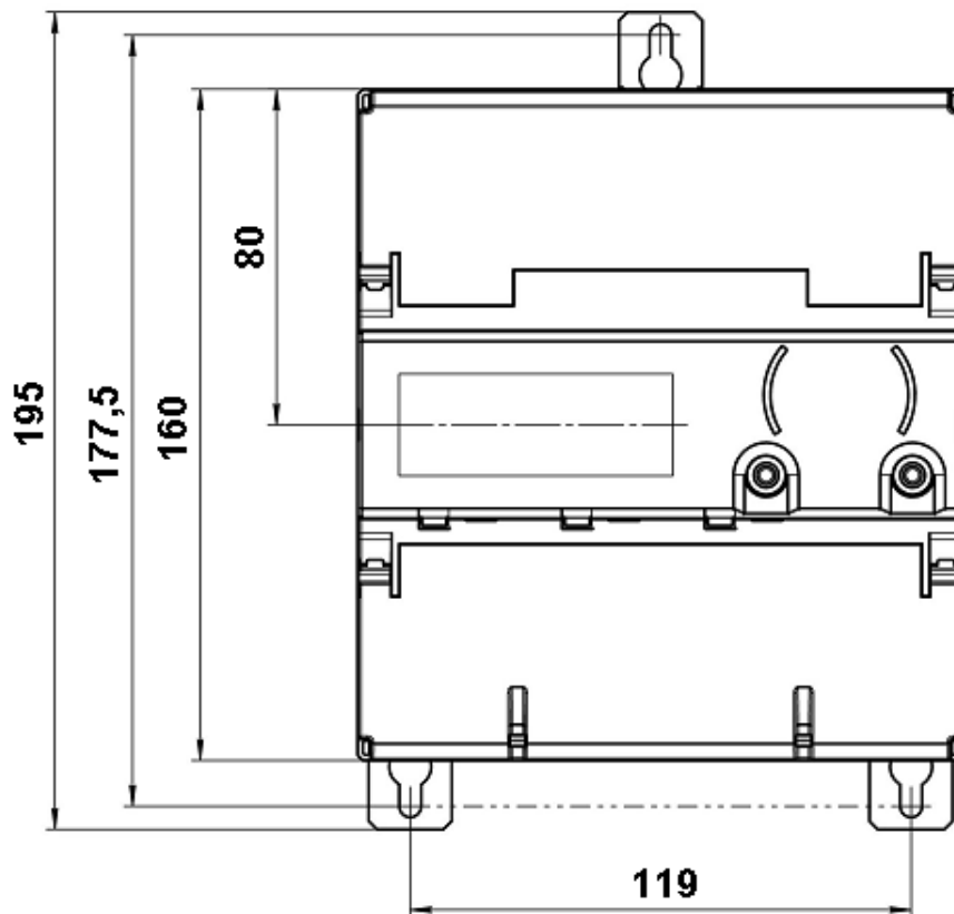
Рисунок А.3 – Крепежные размеры для крепления на стену счетчика Меркурий 350Х
