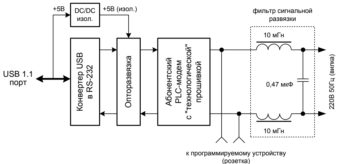
Рисунок 2. Блок-схема ТМ.
